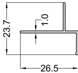
NO : 94-980 0.135 Kg.m.
