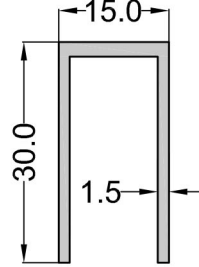
NO : 94-1624 0,310 Kg.m.
