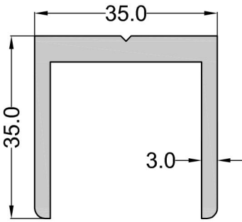
NO : 94-599 0,610 Kg.m.
