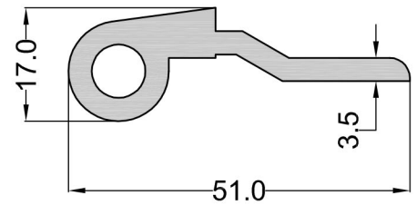
NO : 94-604 0.800 Kg.m.
