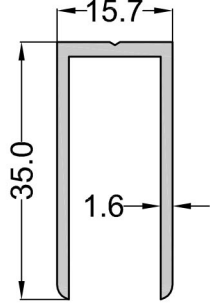
NO : 94-598 0.365 Kg.m.
